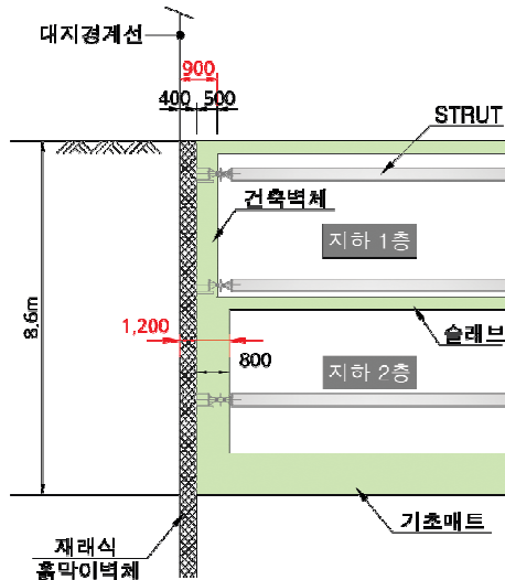
(a) 재래식 흙막이 공법 + 건축영구벽체
