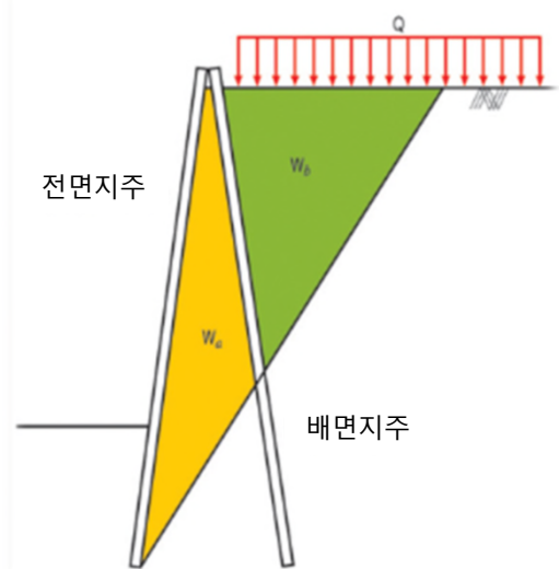
지주식 흙막이 토압 개념도
